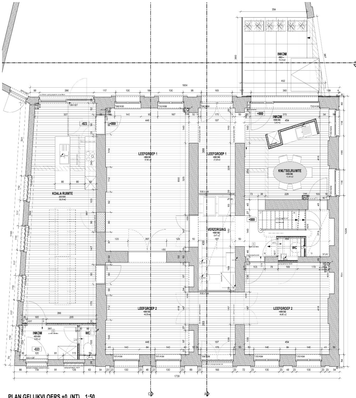
PLAN GELIJKVLOERS +0 (NT) _ 1:50
