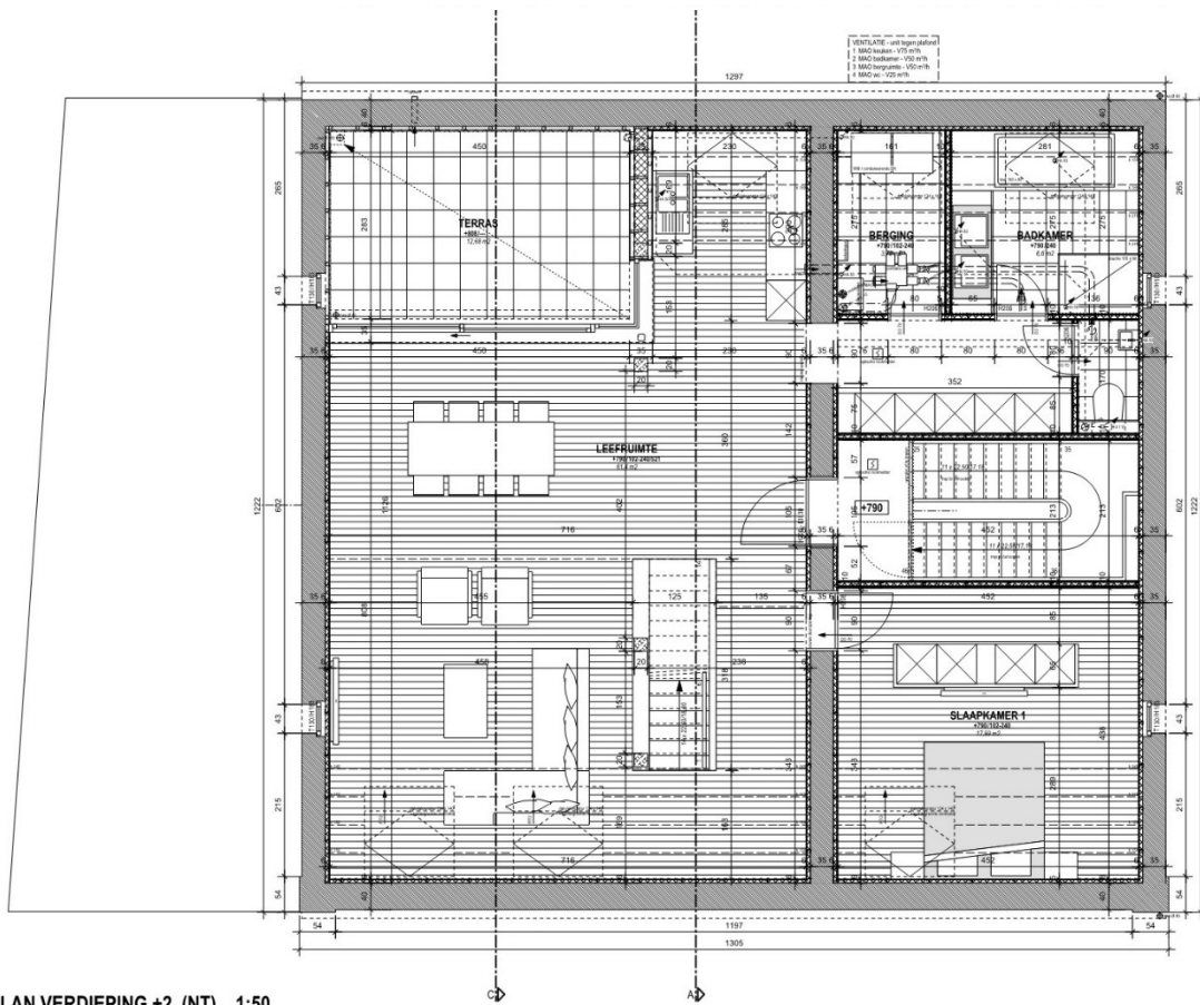
PLAN VERDIEPING +2 (NT) _ 1:50
